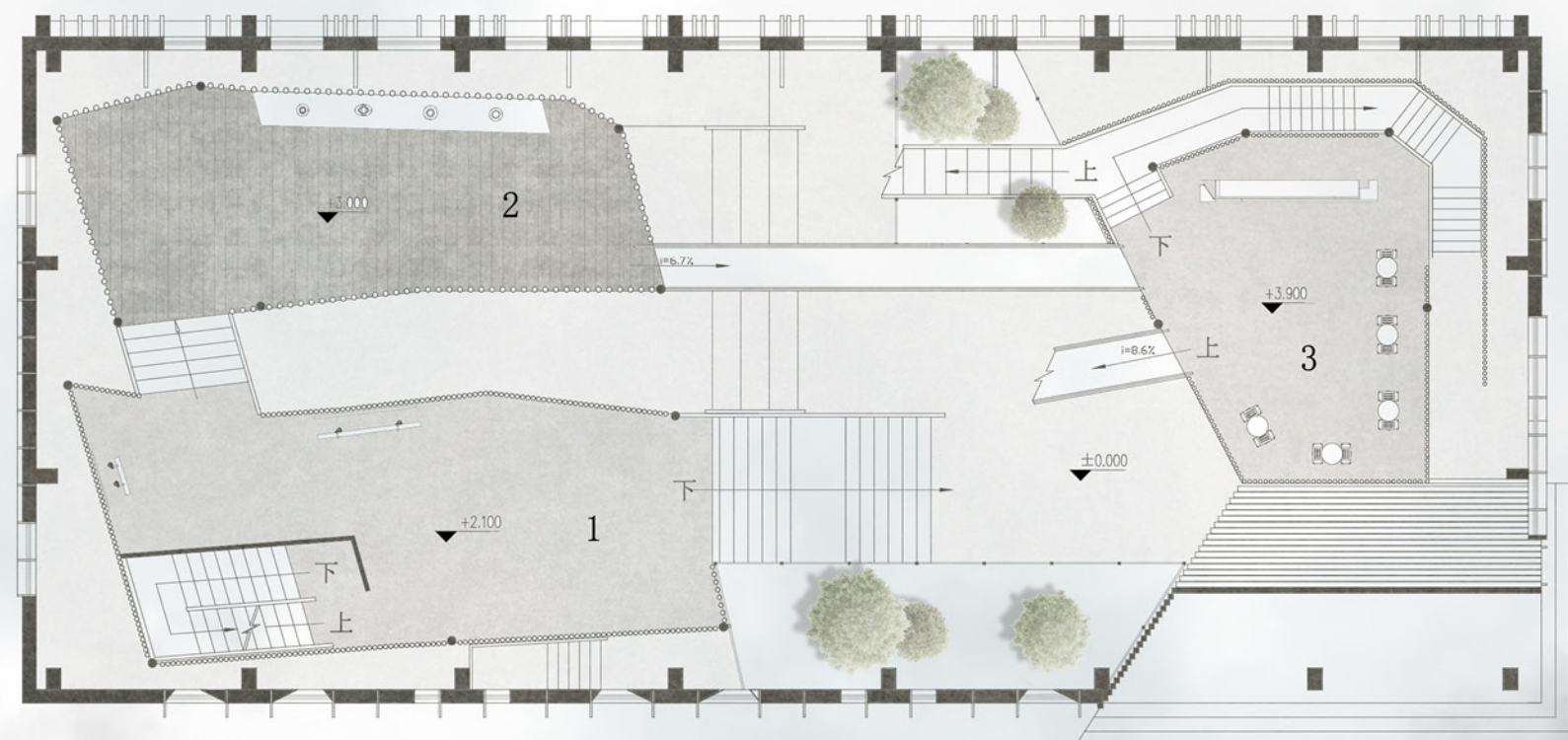
二层平面图 SECOND FLOOR PLAN
