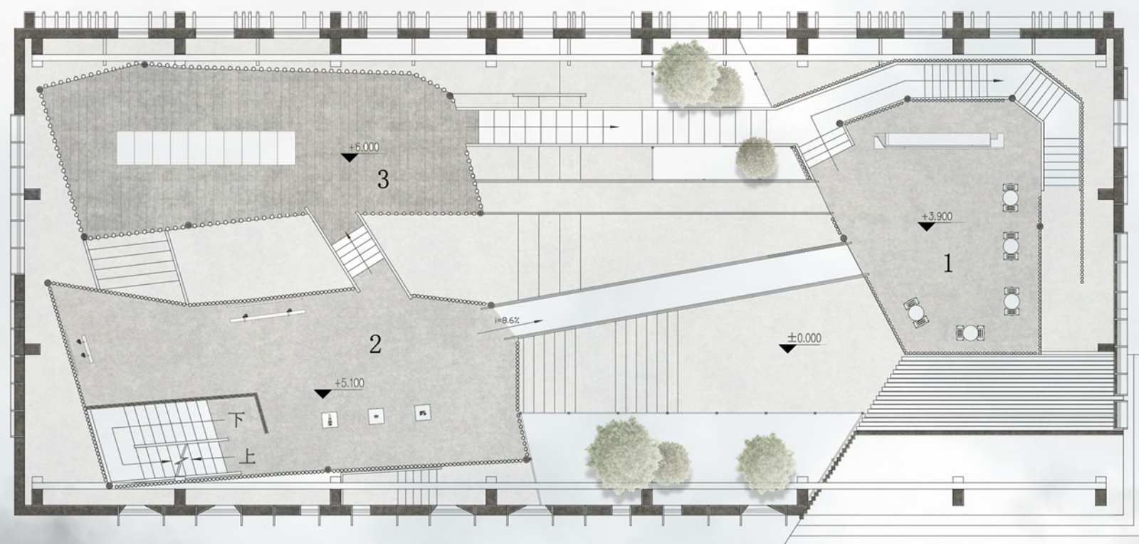
三层平面图 THIRD FLOOR PLAN
